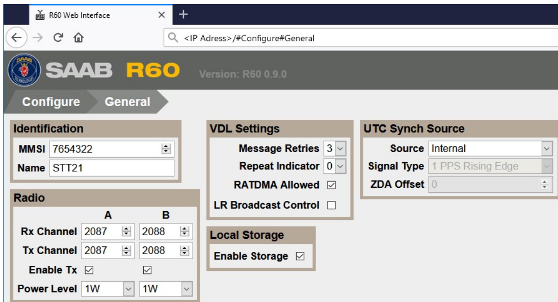
Figura 5-4 Interfaz de configuración
